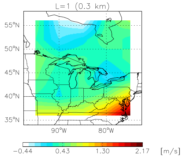
GCAP VWND Jul 1999 – Jul 2001
