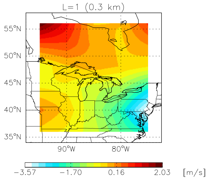
GCAP UWND Oct 1999 – Oct 2001
