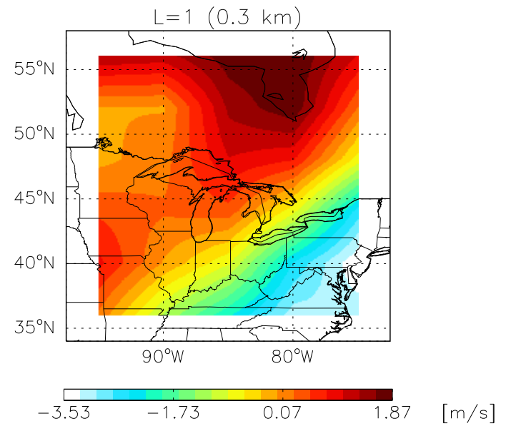
GCAP VWND Oct 1999 – Oct 2001
